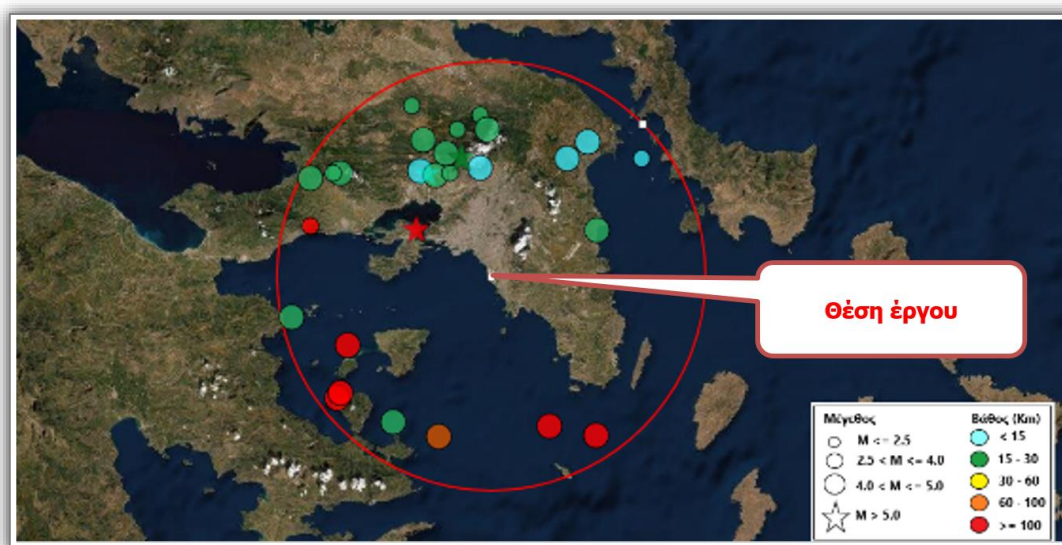
Σχήμα 3-1: Σεισμική Δραστηριότητα σε ακτίνα 50km από Μητροπολιτικό Πόλο (1964-2022, Ms>4,0 Richter). Πηγή: https://www.gein.noa.gr/ypiresies-proionta/vasi-anazitisis/
